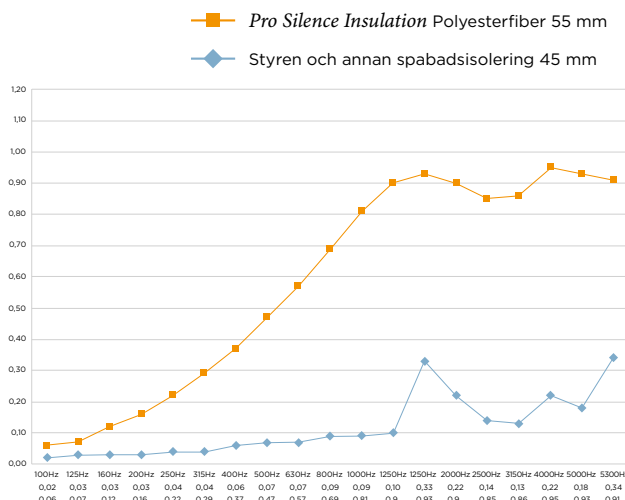
Grafen visar ljudabsorption vid olika frekvenser, ju högre kurva – desto bättre ljudabsorption.
